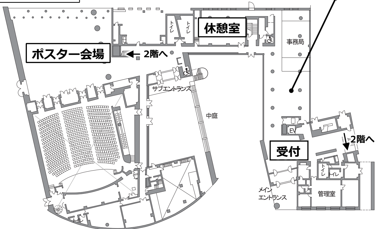
1階配置図
